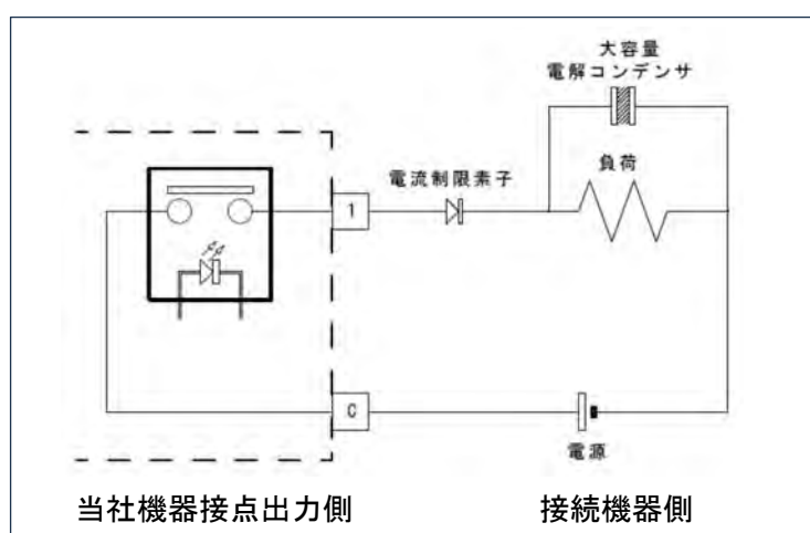
【図7】突入電流制限例
