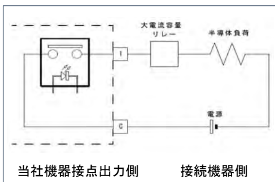
【図5】大電流容量リレーによる保護例
