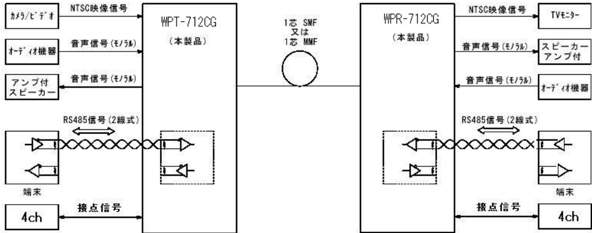
図1 接続構成
