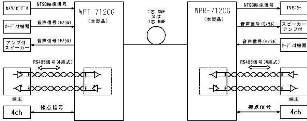
図3 接続構成
