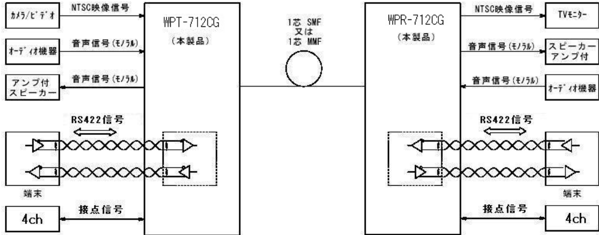
図5 接続構成
