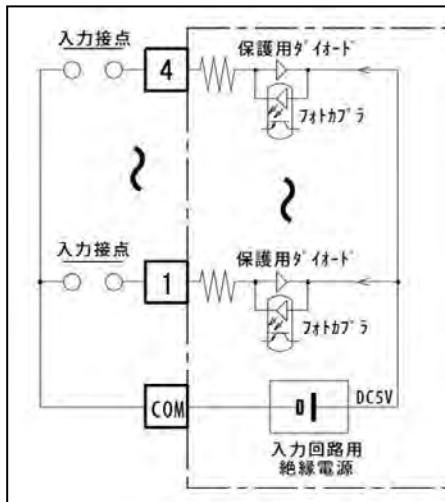
入力構成
