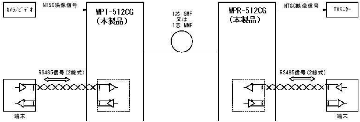
図1 接続構成
