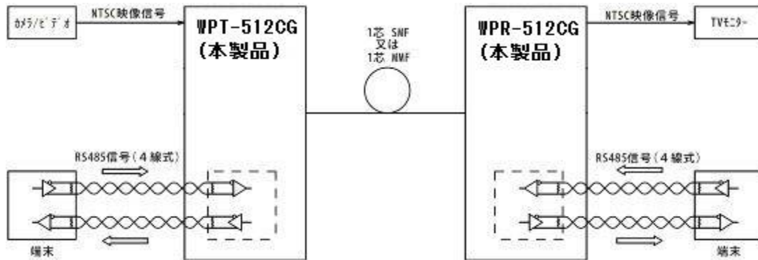
図2 接続構成
