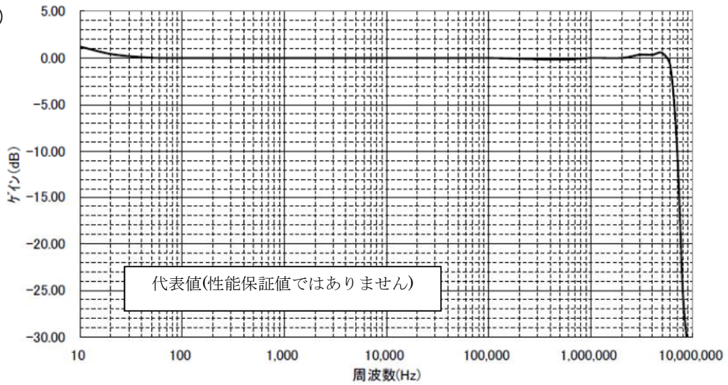
(周波数特性)
