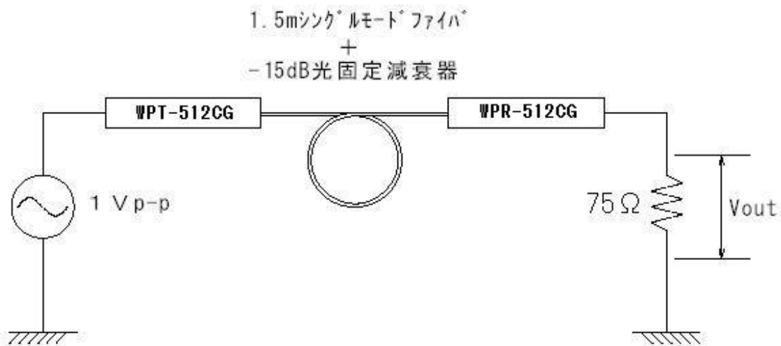
(測定回路)
